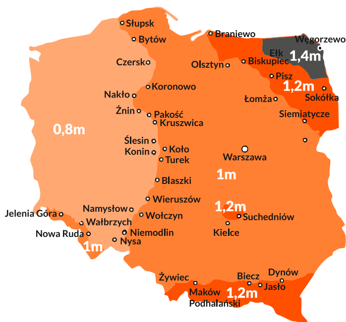
Rys.1 Głębokość przemarzania gruntu wg PN-81/B-03020
